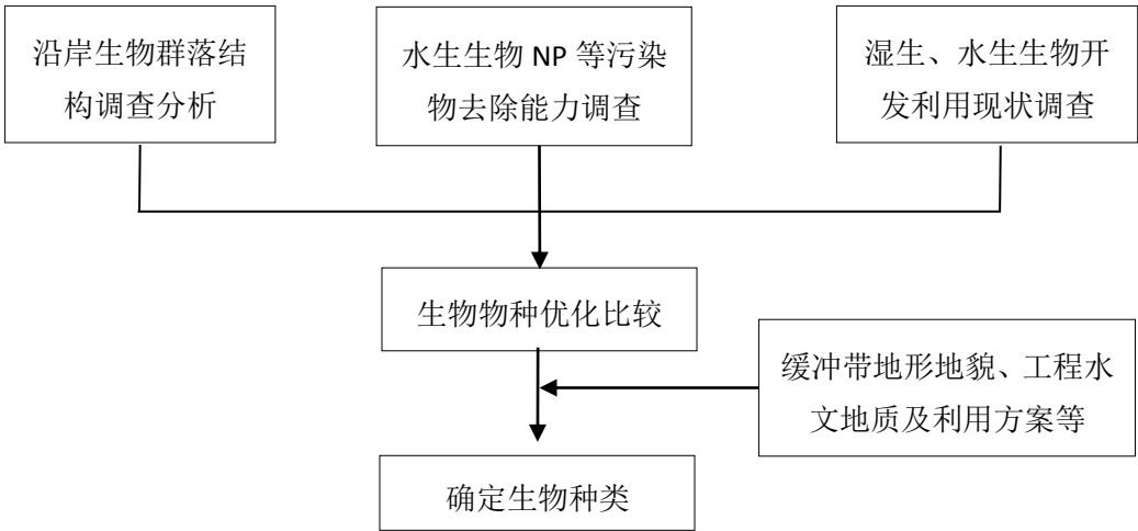
图2 缓冲带植物配置一般流程参考示意图
